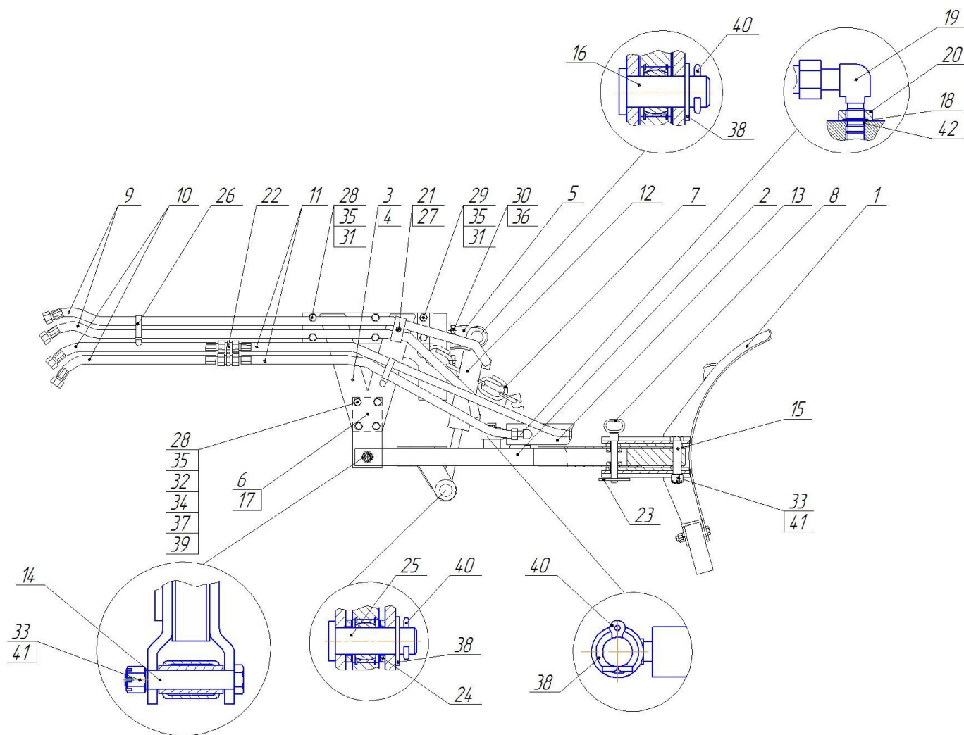
Рис.1 - Общий вид отвала тракторного OT-18/OT-20
