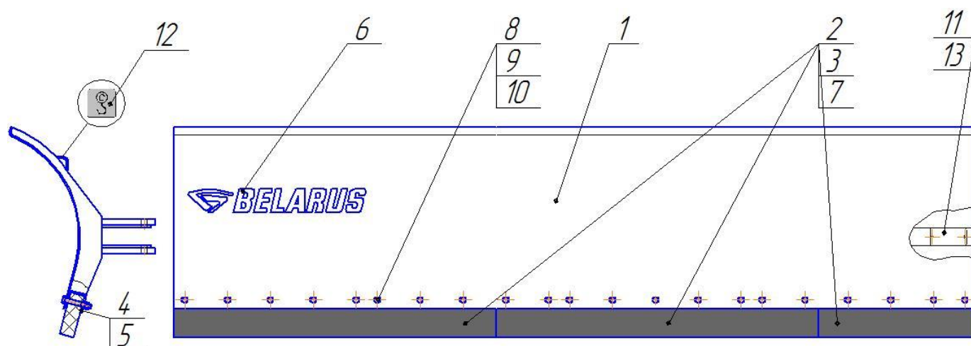
Рис.4 – Отвал OT25-00.00.030
