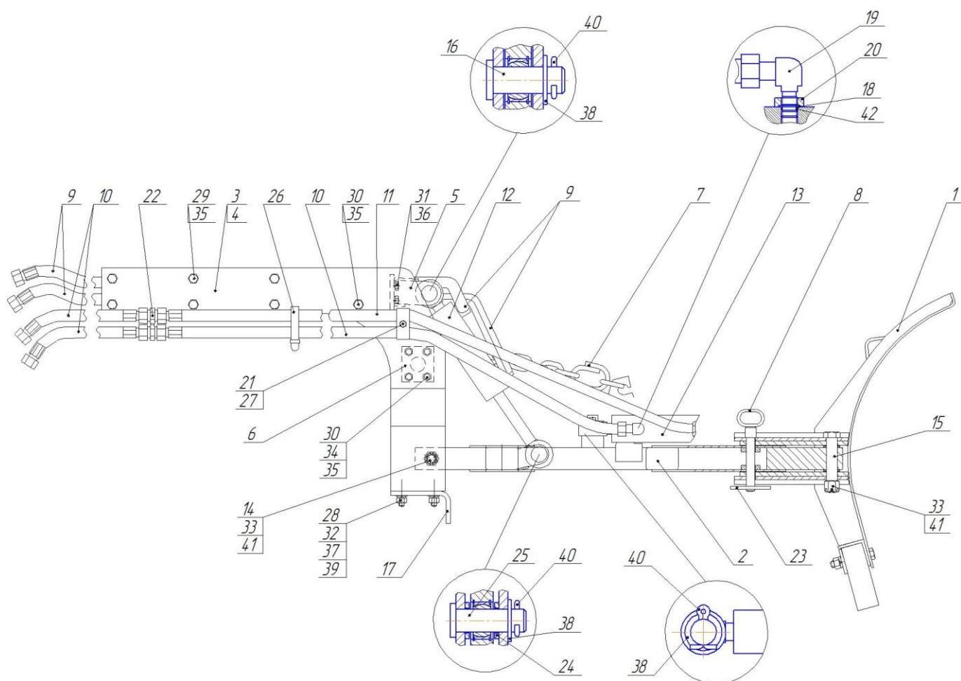
Рис.3 - Общий вид отвала тракторного OT-25
