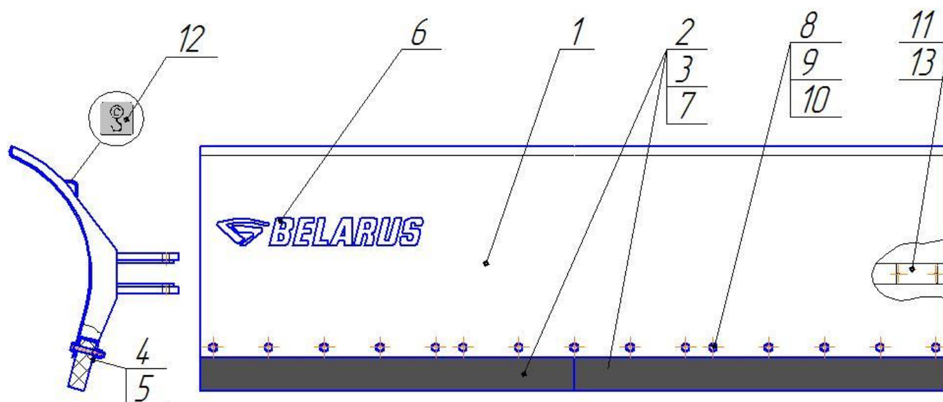
Рис.2 - Отвал OT18/OT20-00.00.030
