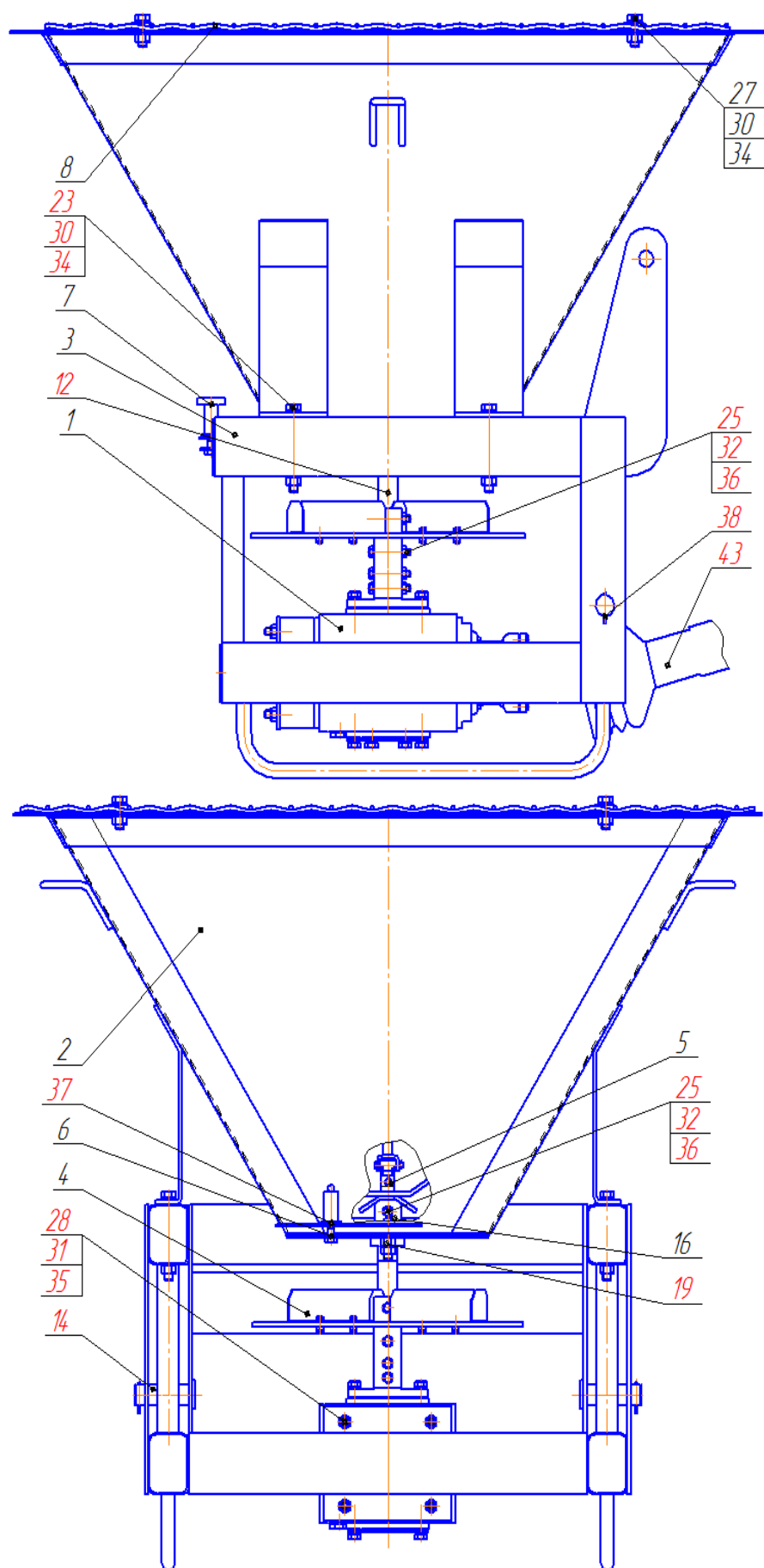
Рис.1 - Общий вид разбрасывателя песка ПР-320
