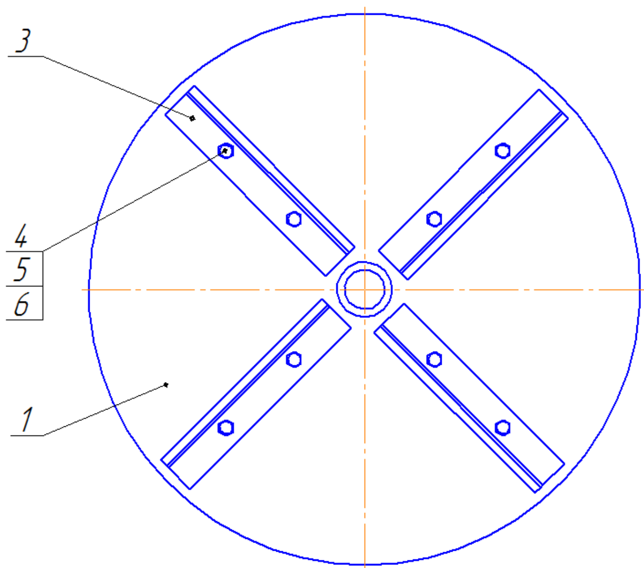
Рис.3 – Опора с диском ПР-320.04.00.000
