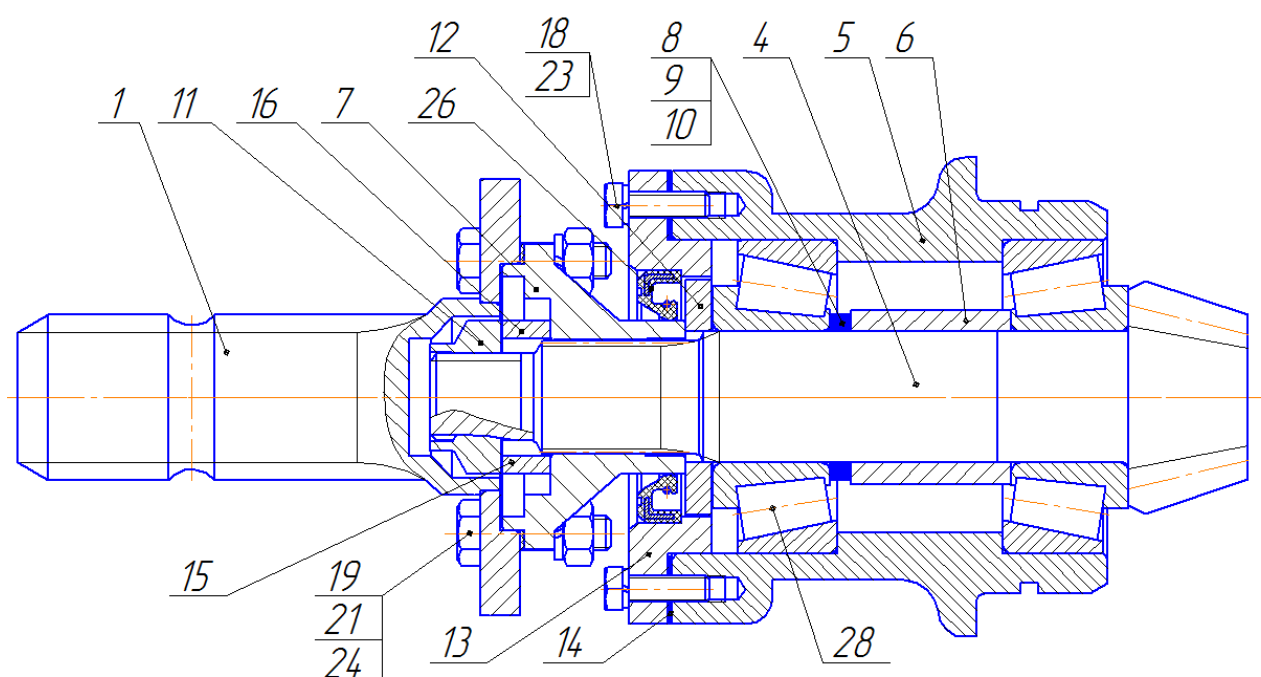
Рис.2.2 – Стакан ПР-320.01.03.000
