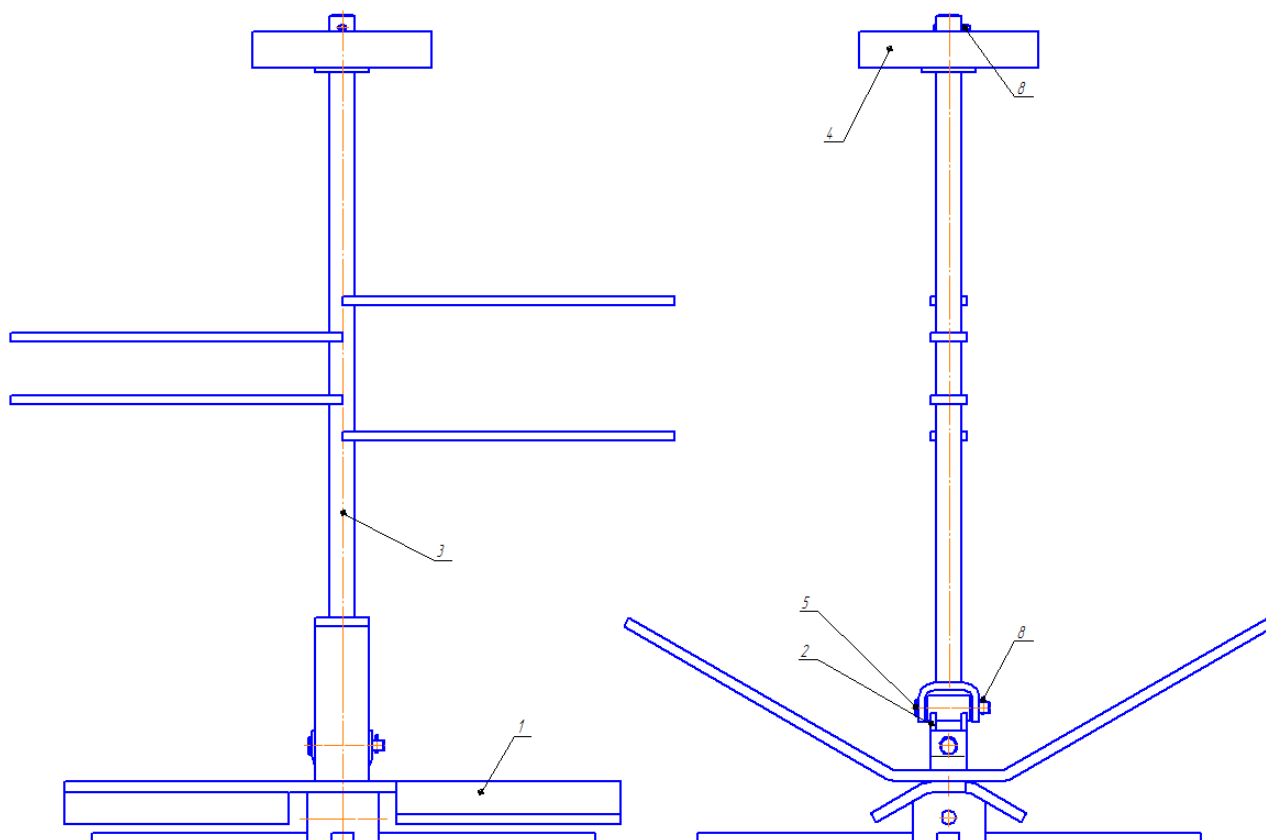
Рис.4 – Рыхлитель ПР-320.05.00.000
